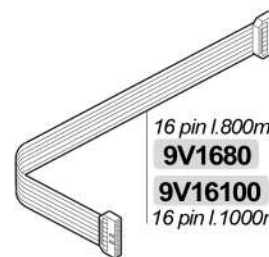
20A 600V IP00 (0-1-2) Generale / General
