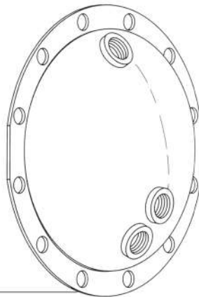
8F150 12 fori EGI / 12 holes EGI
