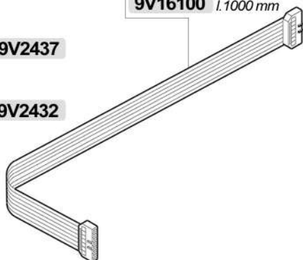
9V1660 l.600 mm 9V1680 l.800 mm 9V16100 l.1000 mm
